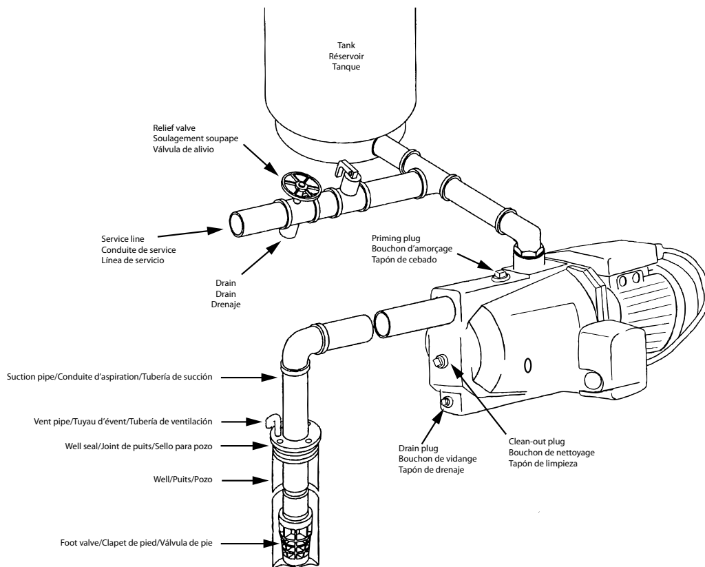
FIGURE 3 SHALLOW WELL (WITH FOOT VALVE) • PUIITS PEU PROFOND (AVEC CLAPET DE PIED) • POZO POCO PROFUNDO (CON VÁLVULA DE ASPIRACIÓN)
