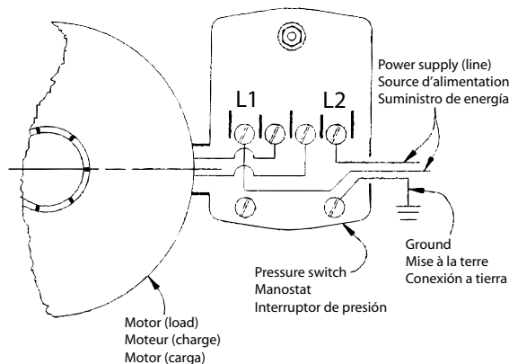
FIGURE 1 ELECTRICAL CONNECTIONS • CONNEXIONS ÉLECTRIQUES • CONEXIONES ELÉCTRICAS
