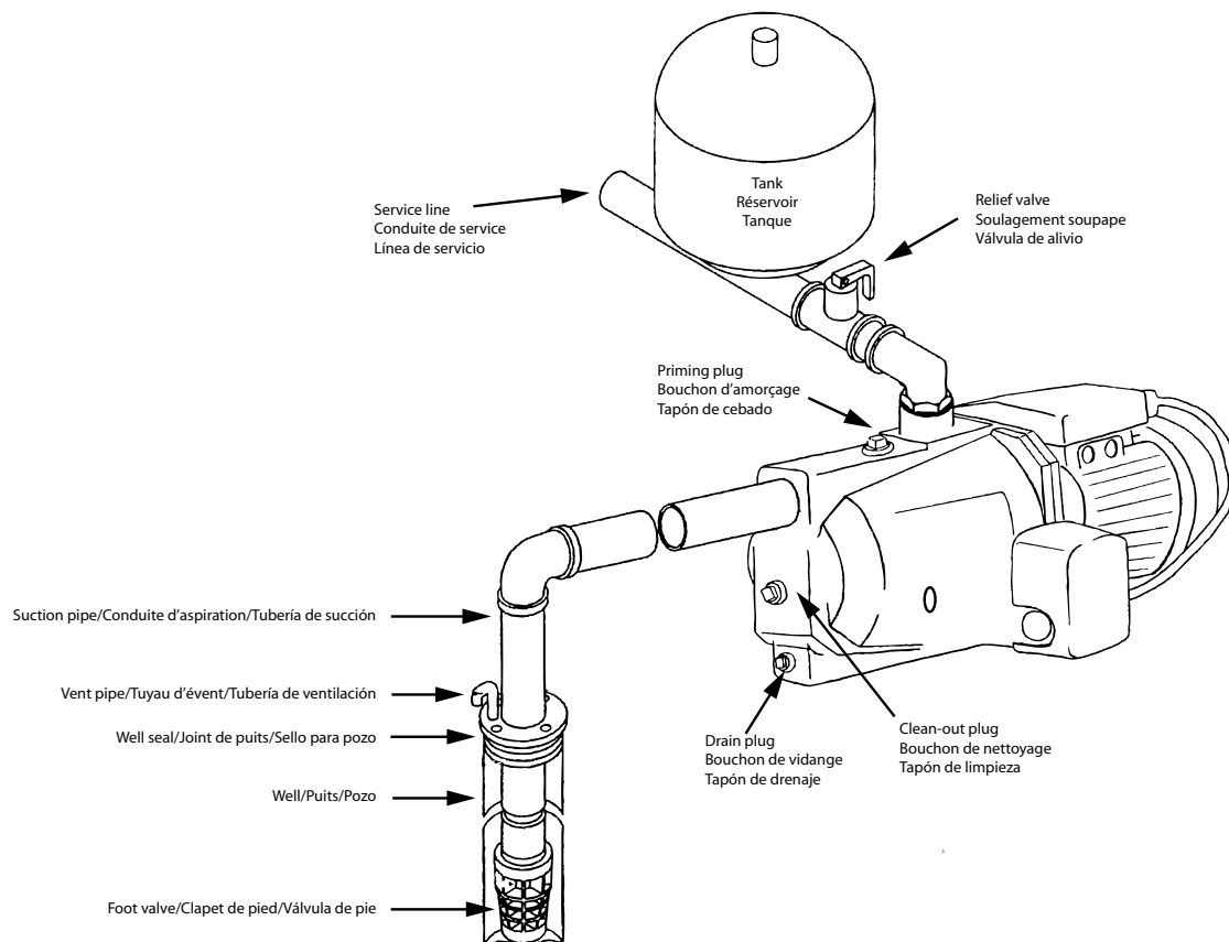
FIGURE 4 SHALLOW WELL - INLINE TANK (WITH FOOT VALVE) • PUIITS PEU PROFOND, RÉSERVOIR EN LIGNE (AVEC CLAPET DE PIED) • POZO POCO PROFUNDO, TANQUE EN LÍNEA (CON VÁLVULA DE ASPIRACIÓN)
